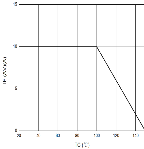
IF(AV) vs TC
