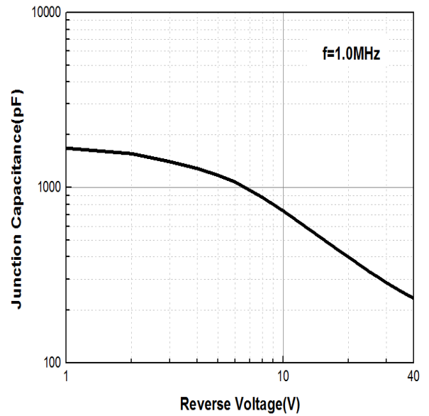
CJ vs VR f=1MHz
