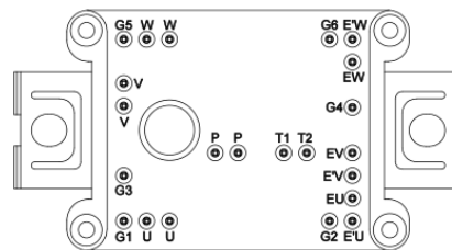
引脚示意图
