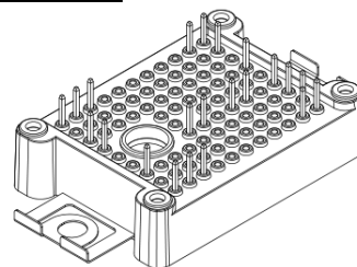
外形示意图
